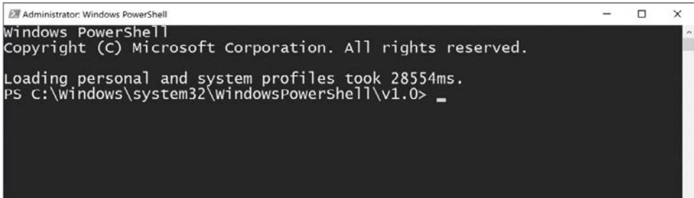
Рис. 1.1. Консоль PowerShell
