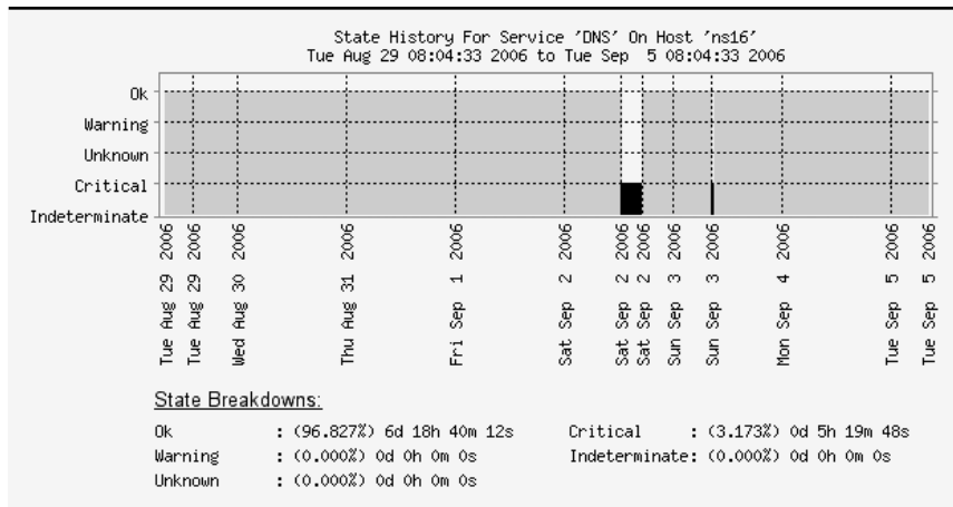
Рис. 19.2. Показатели доступности сервера, отображаемые программой Nagios
