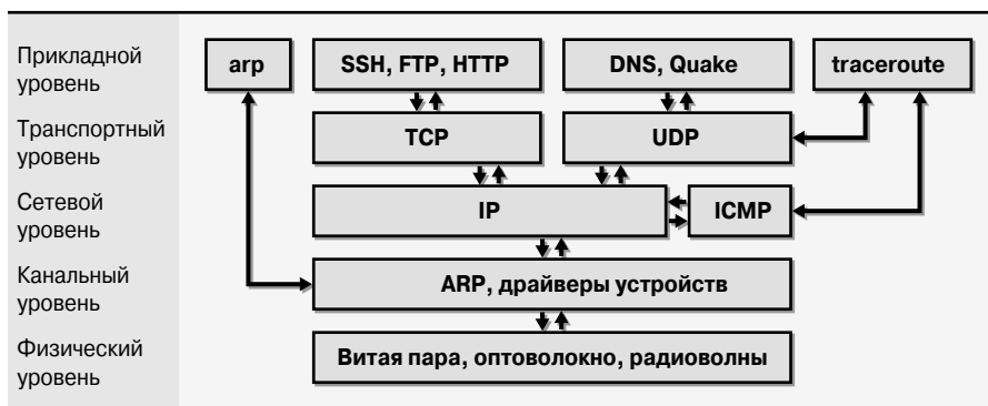
Рис. 12.1. Успешное семейство TCP/IP
