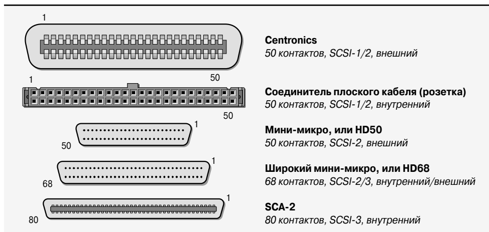
Рис. 7.1. Распространенные SCSI-разъемы (вид спереди; вилка, если не указано иное)
