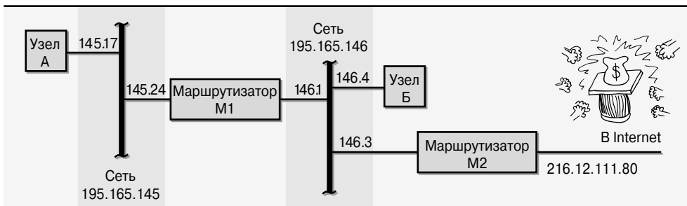
Рис. 13.1. Демонстрационная сеть
