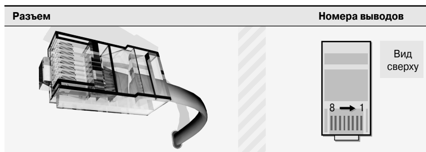
Рис. 27.5. Вилка разъема RJ-45
