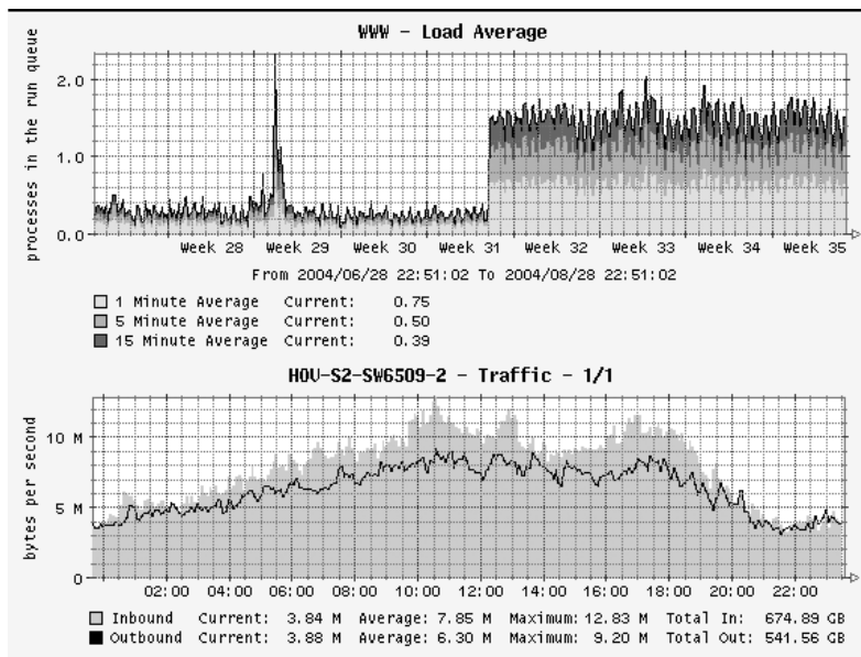
Рис. 19.1. Примеры графиков программы Cacti
