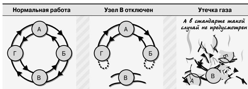
Рис. 14.4. Двойная кольцевая сеть FDDI
