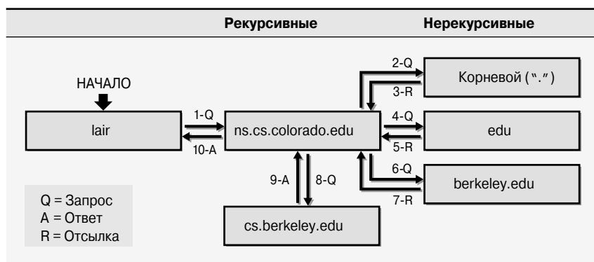
Рис. 15.1. Обработка запроса в DNS
