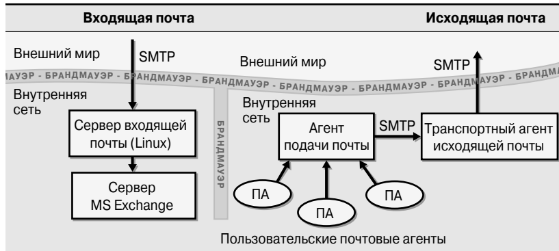
Рис. 18.4. Структура почтовой системы (вариант 2)
