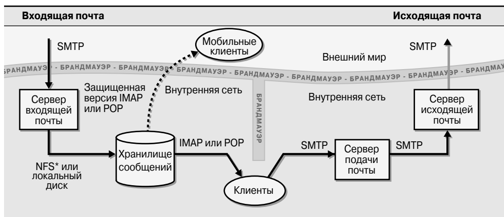
Рис. 18.3. Структура почтовой системы (вариант 1)
