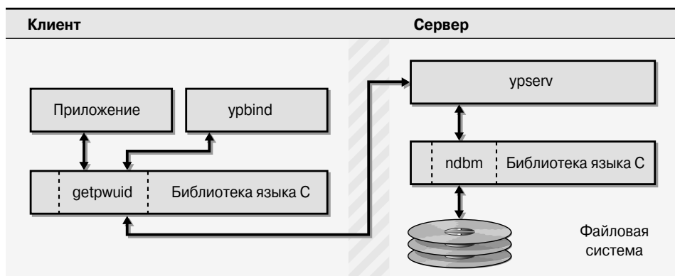
Рис. 17.1. Процедура обработки запросов в NIS
