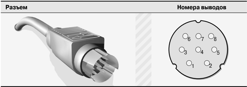
Рис. 27.3. Вилка мини-разъема DIN-8
