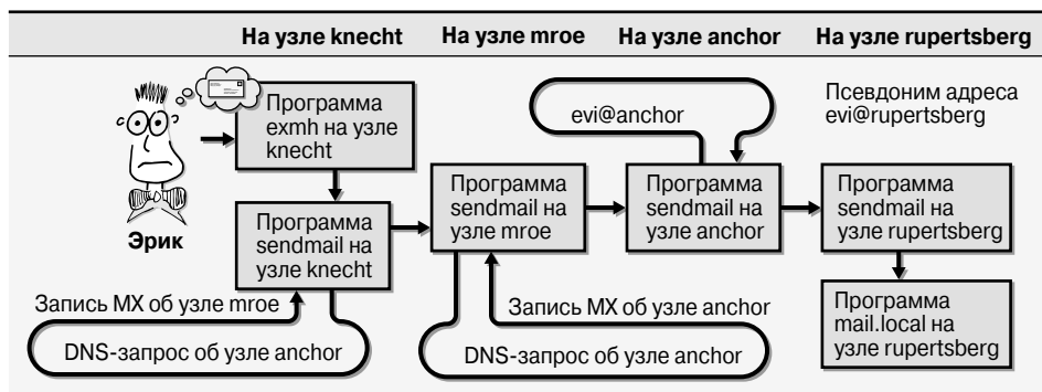
Рис. 18.2. Путь сообщения от Эрика
