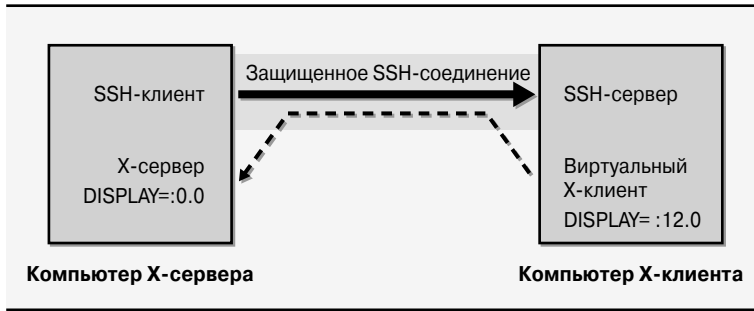
Рис. 22.2. Использование протокола SSH в системе X
