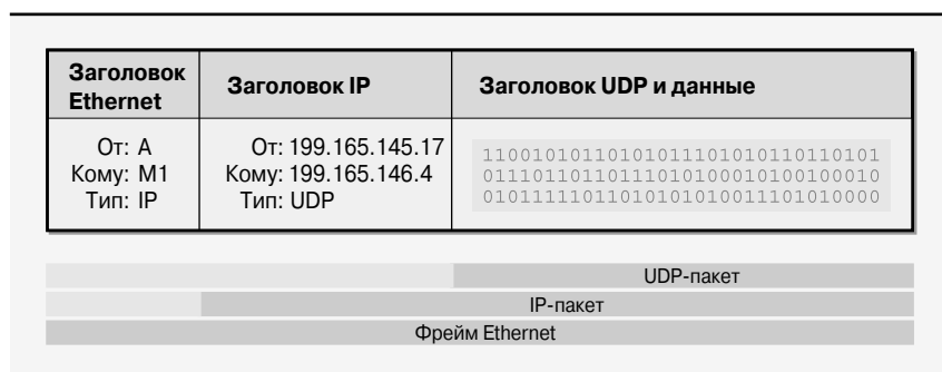
Рис. 13.2. Ethernet-пакет
