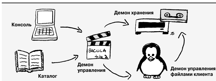
Рис. 9.1. Компоненты системы Bacula и их взаимосвязь
