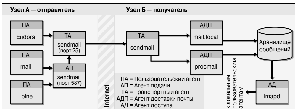
Рис. 18.1. Компоненты почтовой системы
